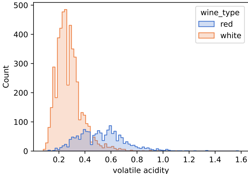
Histograma Incondicional (Bimodalidade) - volatile acidity
